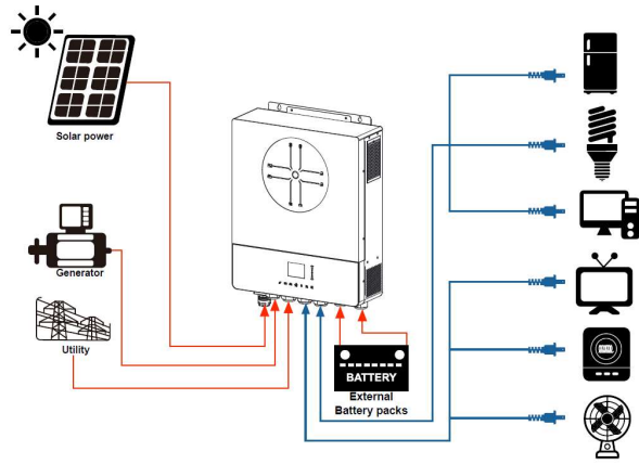
Abbildung 1 Grundlegende Übersicht über hybride PV- Systeme
